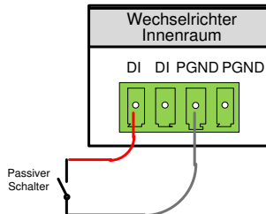
Abb. 5-7 Lokaler Stopp-Kontakt
