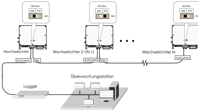
Abb. 5-4 Status Abschlusswiderstände
