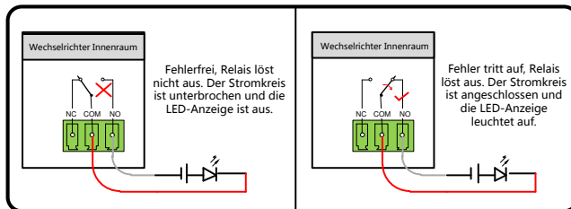
Abb. 5-5 Schließerkontakt
