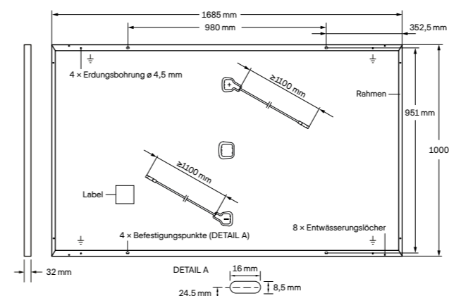
Abb. 1: Außenmaße (in mm) und Komponenten für Q.PEAK DUO-G7, Q.PEAK DUO BLK-G7, Q.PEAK DUO-G7.2 und Q.PEAK DUO BLK-G7.2
