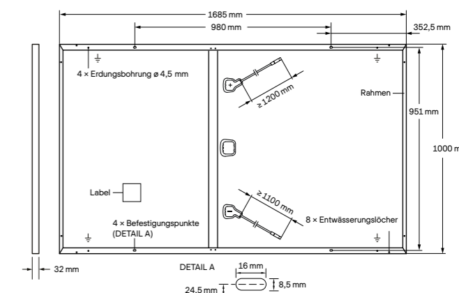
Abb. 2: Außenmaße (in mm) und Komponenten für Q.PEAK DUO-G7.1 und Q.PEAK DUO-G7.3
