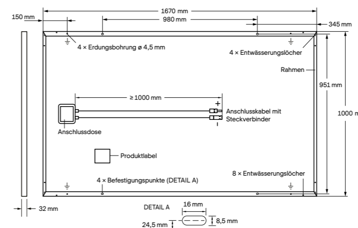
Abb. 1: Außenmaße (in mm) und Komponenten für Q.PEAK-G4.4, Q.PEAK BLK-G4.4 und Q.PEAK-G4.5
