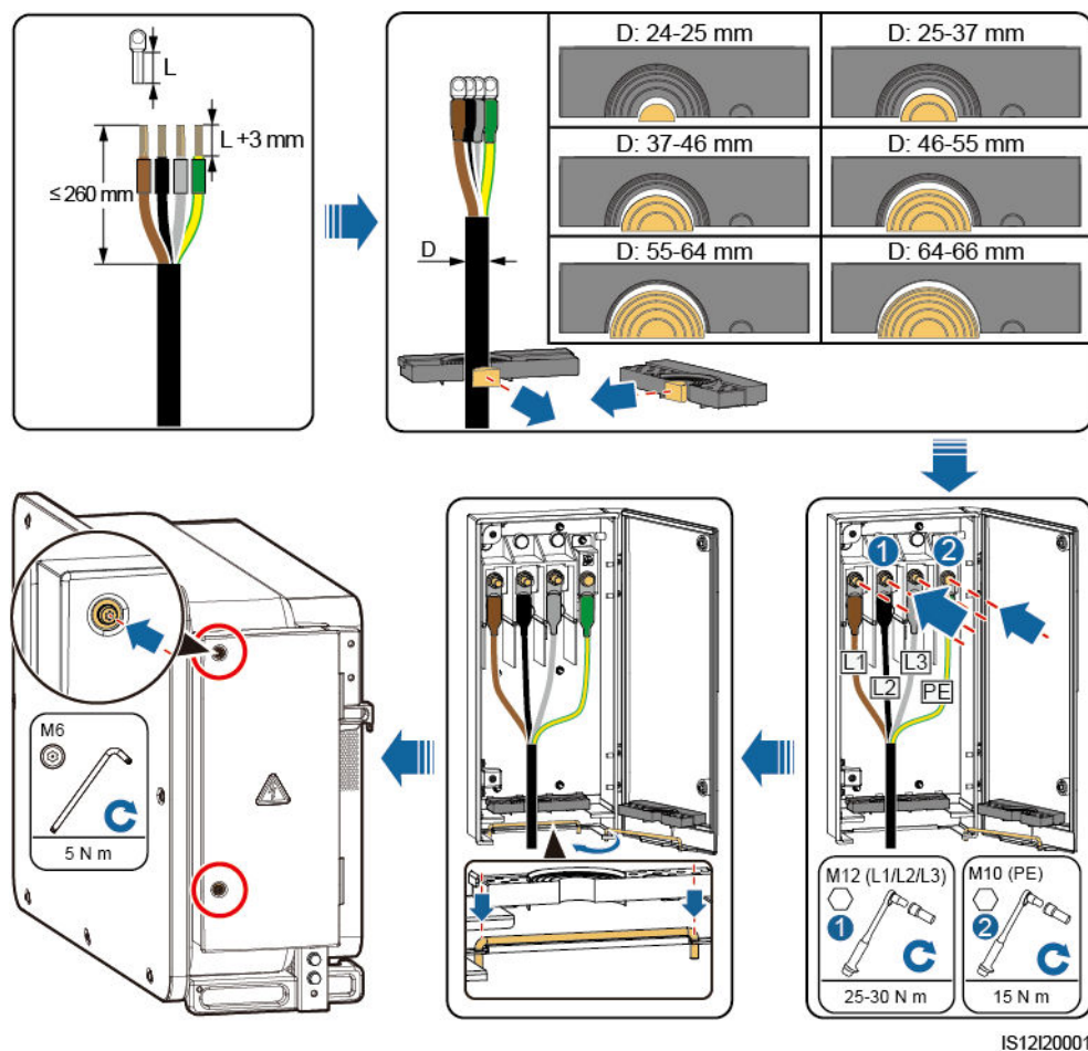
Abbildung 5-16 Verbindungen der mehradrigen Kabel
