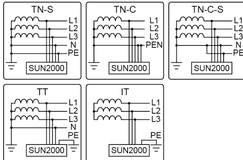
Abbildung 2-5 Unterstützte Stromnetze
