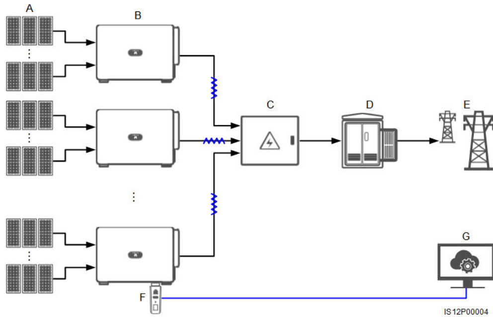
Abbildung 5-4 MBUS-Vernetzung (SDongle)
